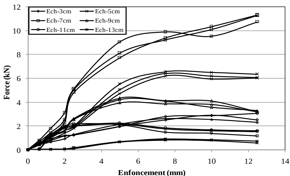
Figure 5. Forces enregistrées durant les essais CBR réalisés sur GCE/SDD.
