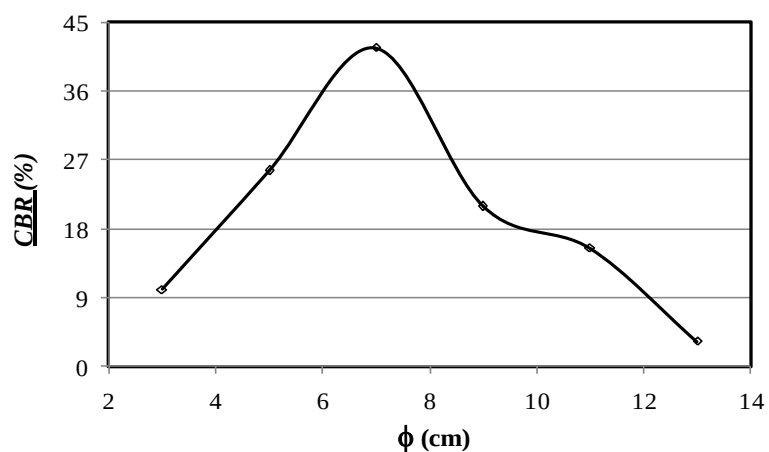
Figure 6: Variation de l'indice CBR en fonction du diamètre des cylindres GTX.
