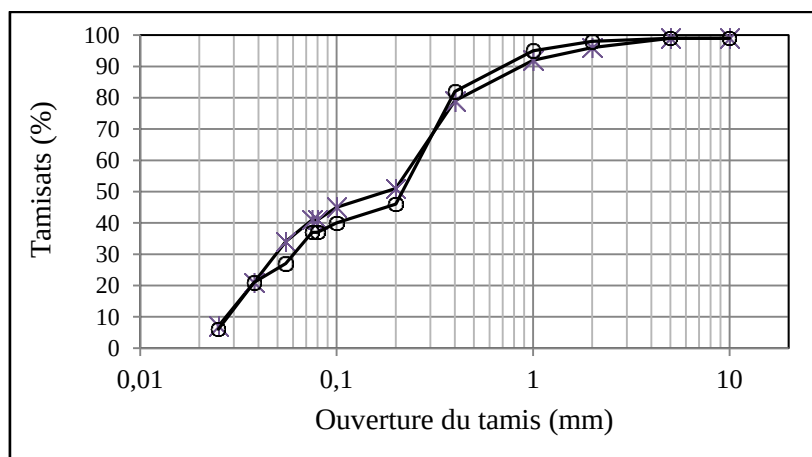
Figure 4: Résultats d'analyses granulométriques sur le tuf.
