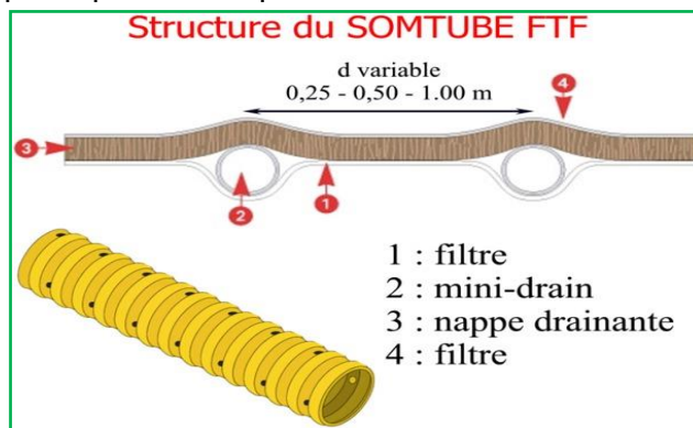
Figure 3. Structure du géocomposite de drainage.
