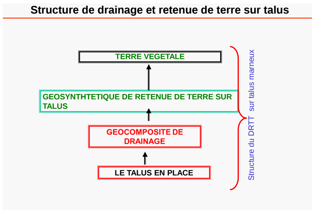
Figure 2. Le dispositif de la solution variante
